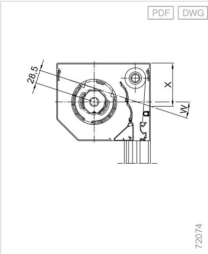
Abgangswinkel Kurbel Typ 1, Linksroller
