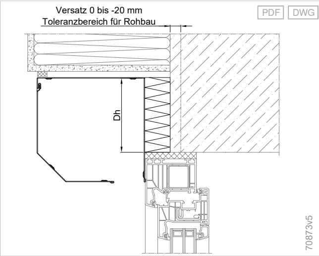
Einbaubeispiel Vorbau-Rollläden mit Sturzdämmung
