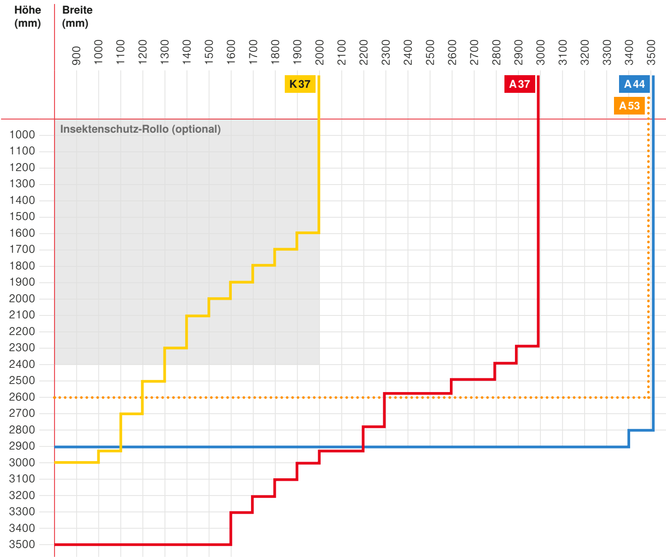
Flächendiagramm Vorbau-Rollläden V6 (Maximale Maße für Einzelflächen)
