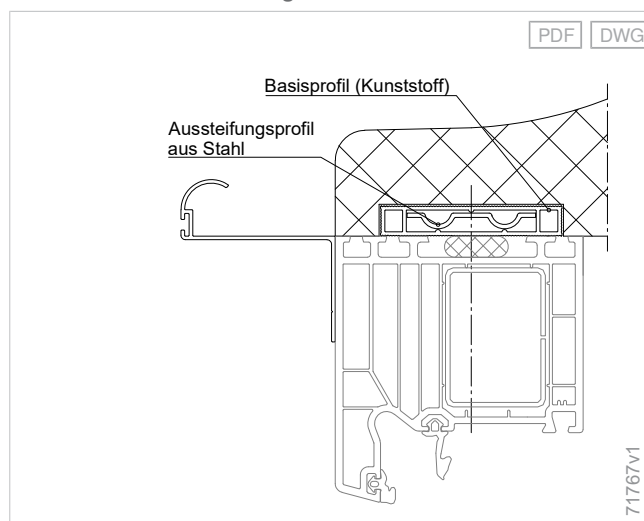
Standard-Fensteranbindung
