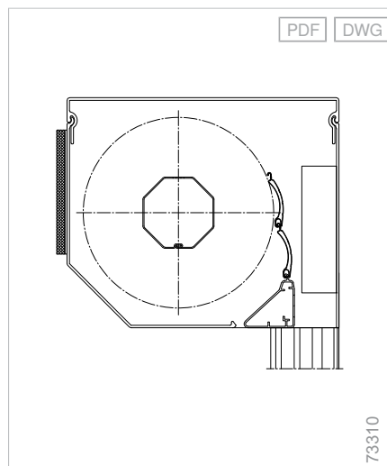
Vorbau-Rollladen V10, Eckig, EWFS SolarKit
