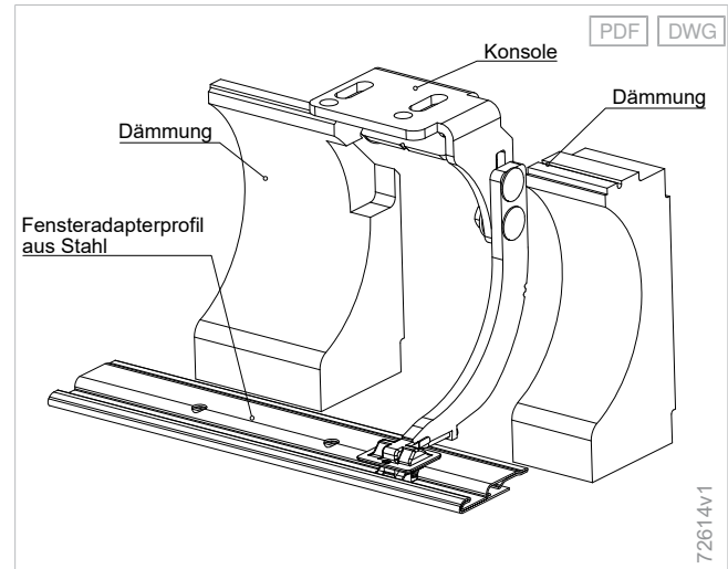
Statikkonsole
