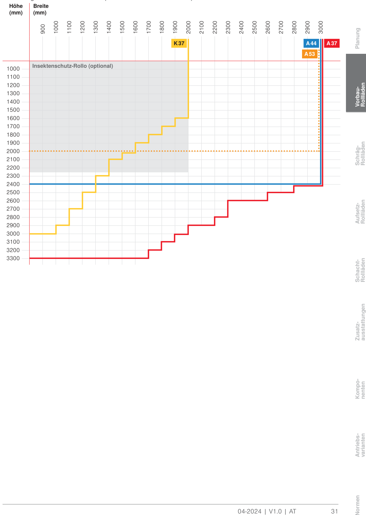
Flächendiagramm Vorbau-Rollläden V4 (Maximale Maße für Einzelflächen)
