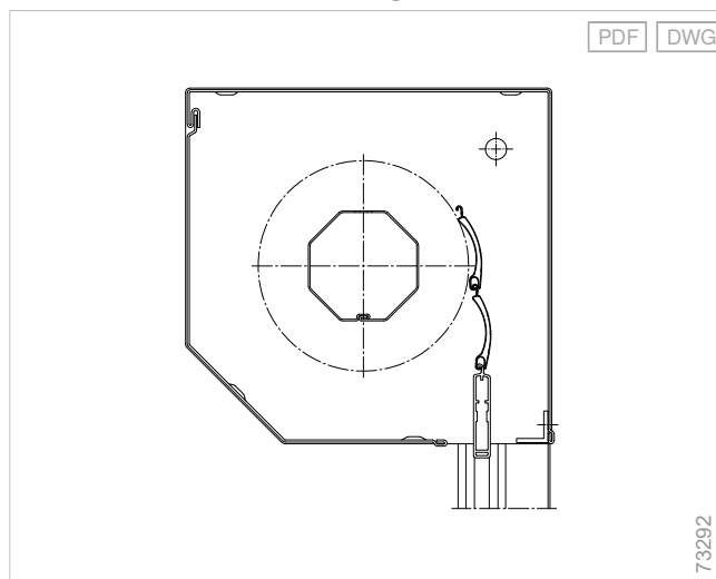
Vorbau-Rollladen, Auslassschlitz geschlossen
